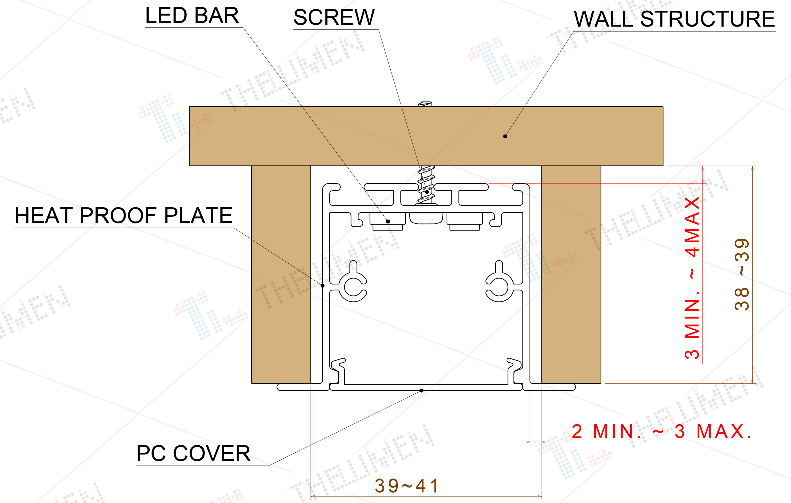
조립 부품 명칭
